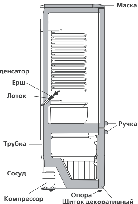
Рисунок 6 — Схема слива талой воды из холодильной камеры
