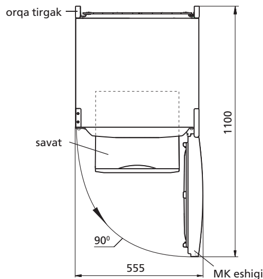
2 rasm — Sovutgich (tepadan ko'rinish)
