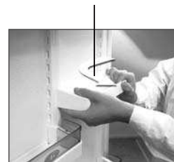
Рисунок 4 — Схема перенавески барьера-полки
