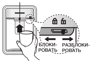
Рычаг диспенсера
